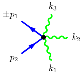
(d) Three Gluon - Quark Vertex. (A.48) on page 128.
